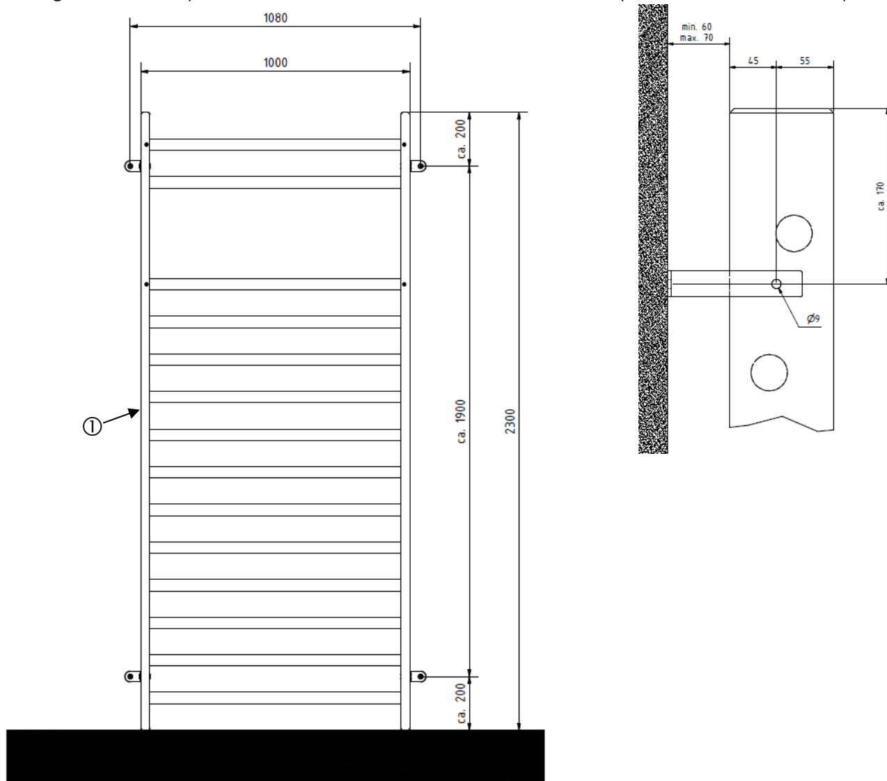
Abbildung 3: empfohlene Bohrbilder und Maßangaben
