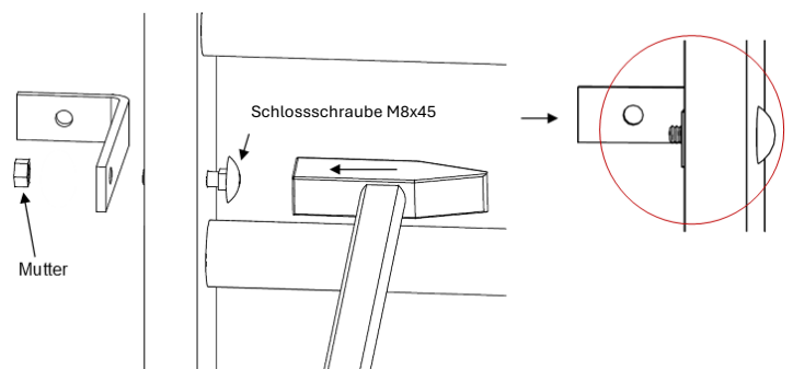
Abbildung 2: Befestigen des Winkels an der Wange
